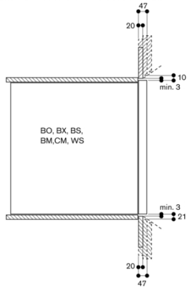
Ventilasjonsareal ved dørkantene oppe/nede
